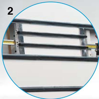
Possibilità base di appoggio di solo ruote frenate o folli. Possibility to get base bottom on braking or free rollers. Posibilidad base de apoyo abajo con ruedas frenadas o libres. Possibilité d'avoir plan d'appui sur rouleaux freinés ou non freinés.
