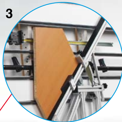
Base di appoggio su blocchi e ruote a scomparsa. Base with supports and retractable rollers. Base de apoyo con soportes y ruedas retractiles. Base d'appui avec sabots et rouleaux escamotables.
